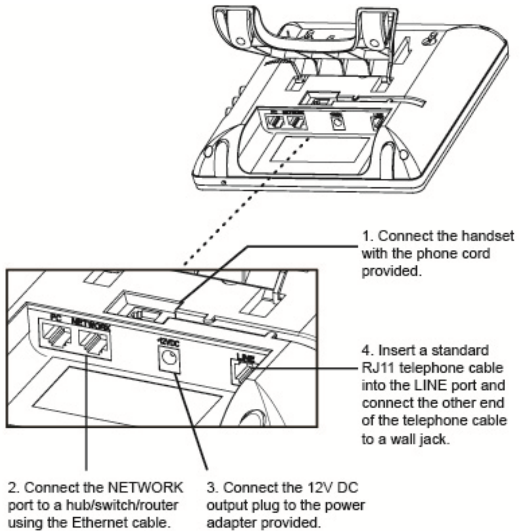
Figura 5: Conectando el GXV3140
